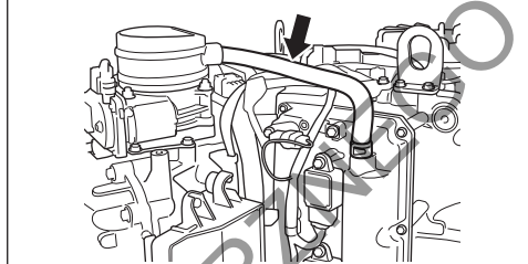
przewód odpowietrzający
