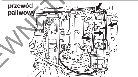
przewód paliwowy
